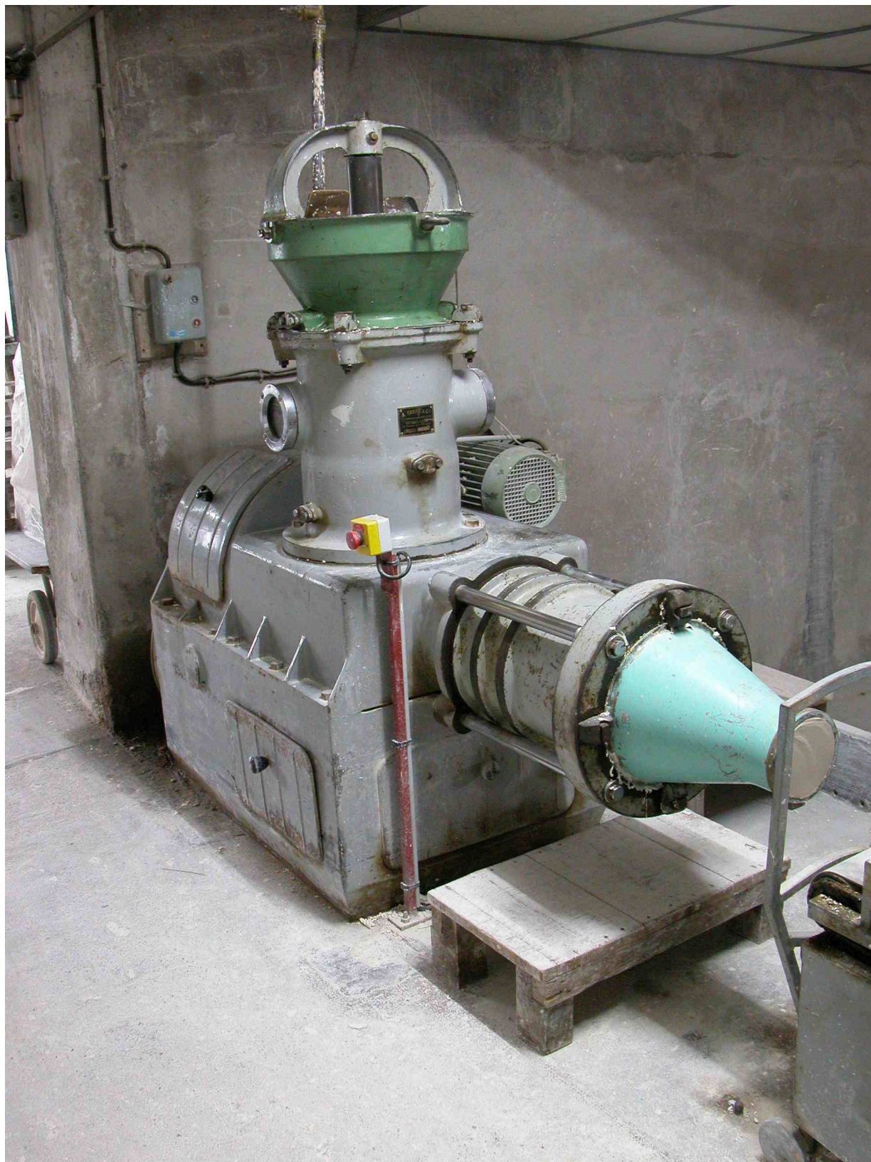
Fig.1 Vue générale de la désaéreuse.
