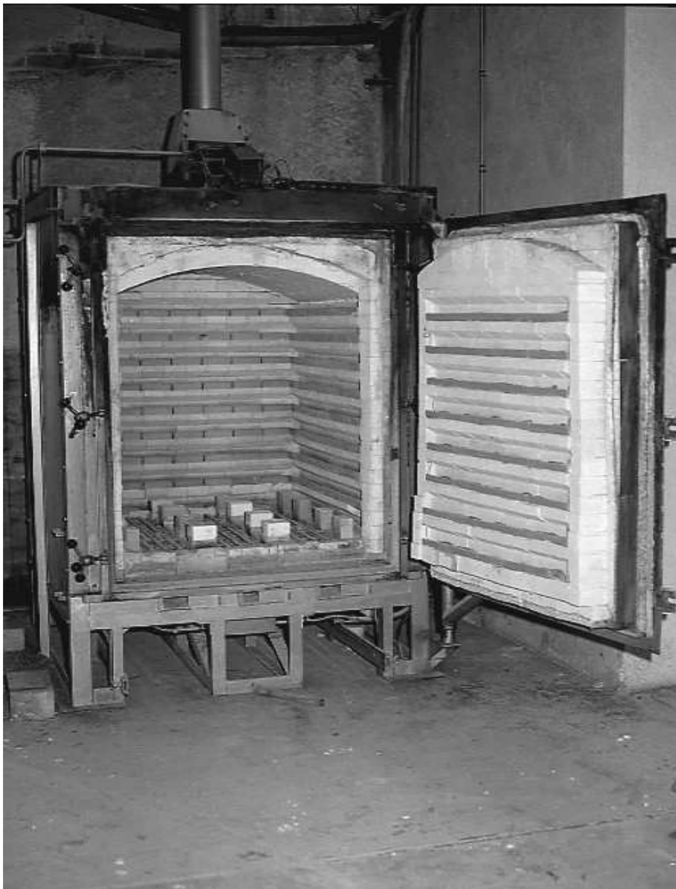
Fig.1 Four-cellule pour la cuisson de dégourdi, porte ouverte.
